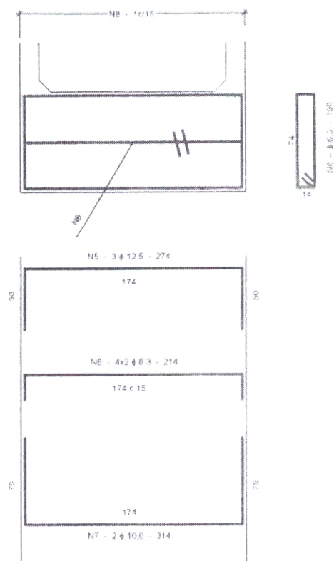
VIGA DE TOPO DA LAJE INFERIOR
