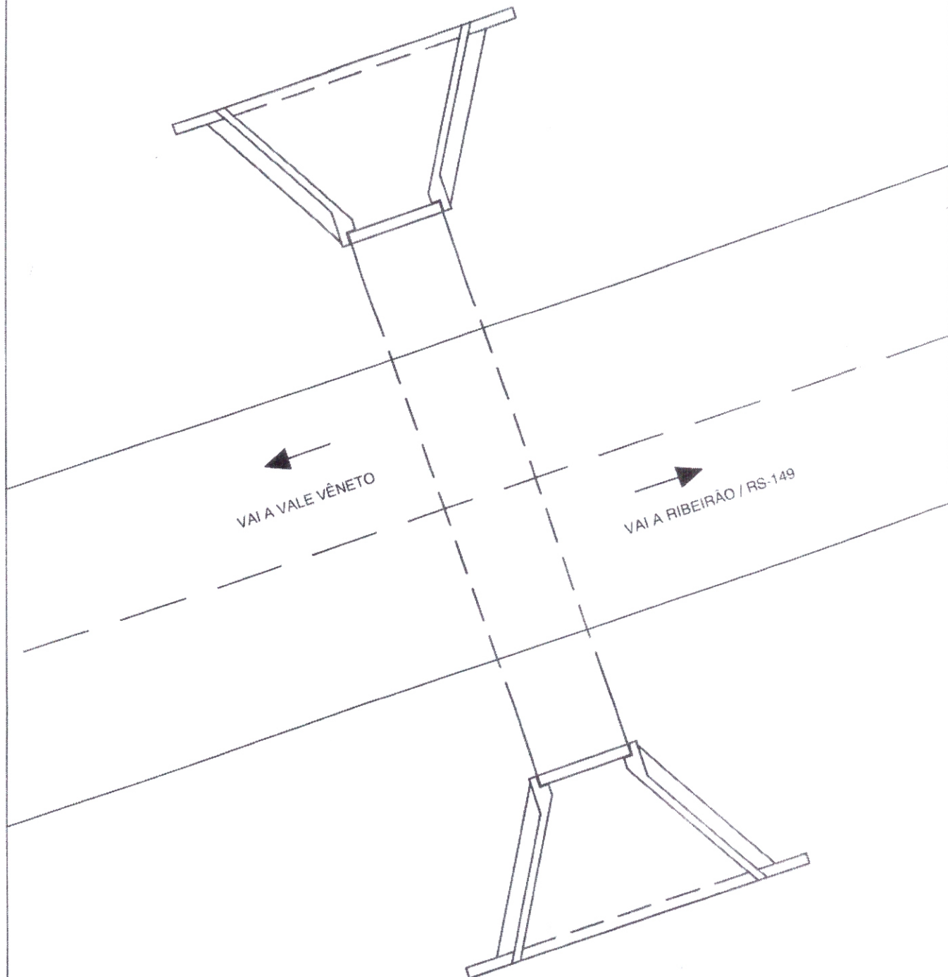
GALERIA PRÉ-MOLDADA DE CONCRETO - SITUAÇÃO
