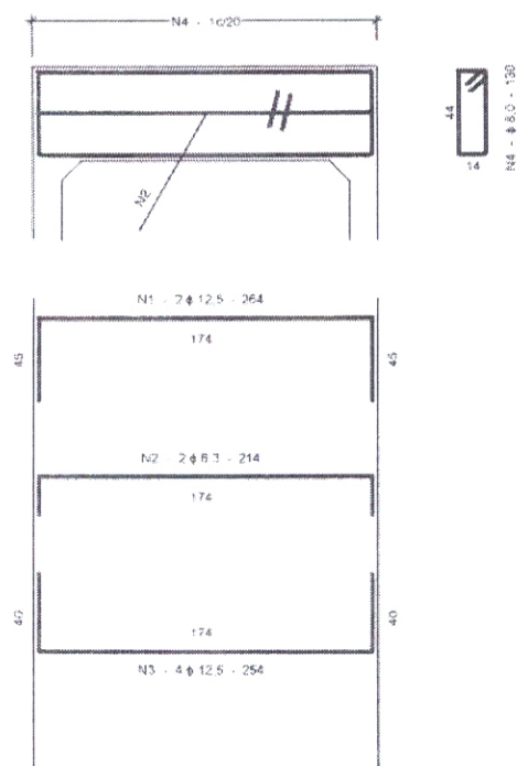
VIGA DE TOPO DA LAJE SUPERIOR
